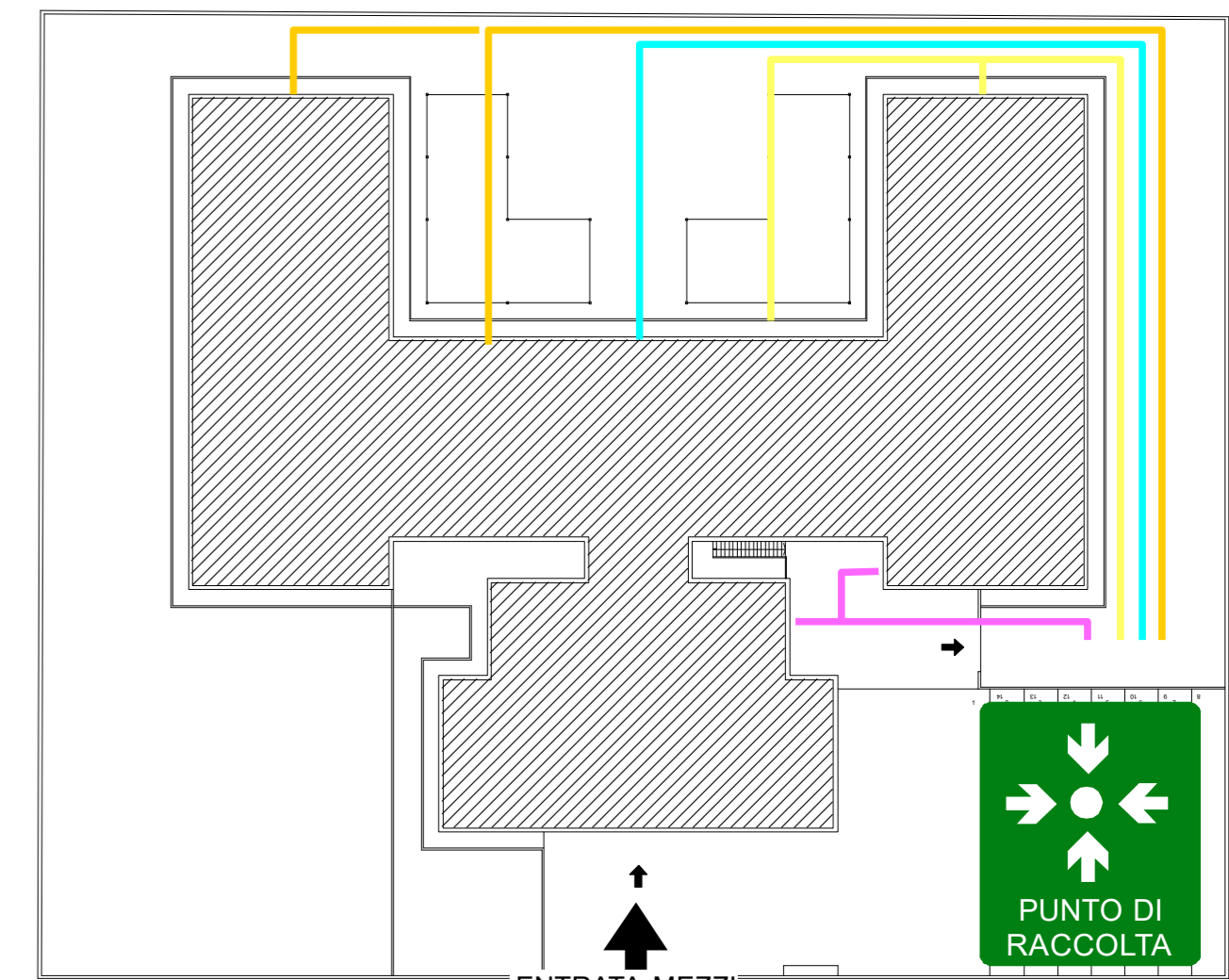
PLANIMETRIA GENERALE
